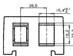
Modular Jack Kat. 5 AMP-Modular Jack System (8polig geschirmt Kategorie 5) (siehe Übersicht)
