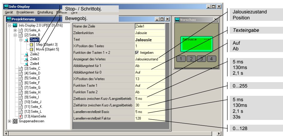
Abb. 12-10 Beispiel Jalousie
