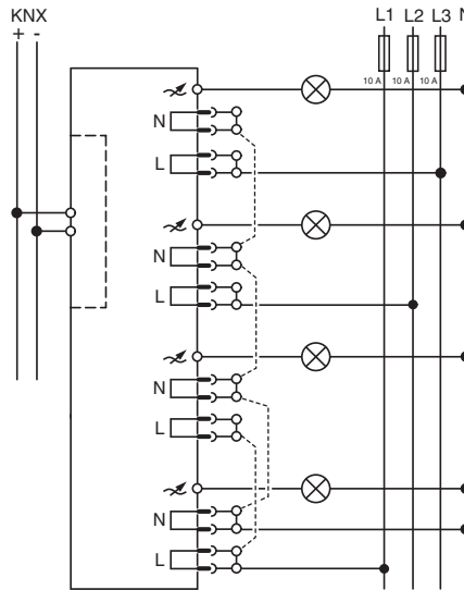
Anschlussdiagramm 4fach Aktor (Beispiel)
