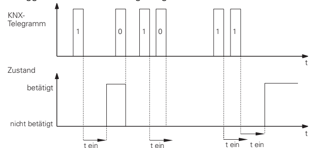
Retriggerbare Einschaltverzögerung
