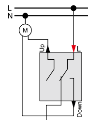
Rolladenschalter mit Zusatzkontakt MEG3714-0000
