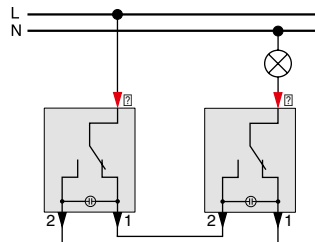
Aus/Wechselschalter mit Orientierungslicht MEG3136-0000
