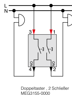
Doppeltaster, 2 Schließer
