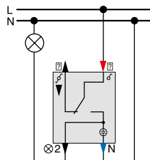
Aus/Wechsel-Kontrollschalter MEG3106-0000
