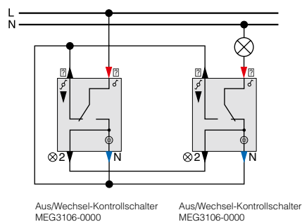
Wechsel-Kontrollschalter als Wechselschalter mit Orientierungslicht
