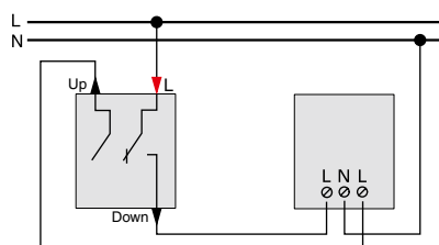
Pollladenschalter MEG3715-0000
