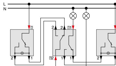
Aus/Wechselschalter mit Orientierungslicht MEG3136-0000
