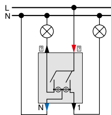
Serien-Kontrollschalter MEG3105-0000
