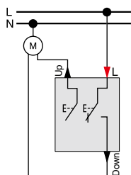
Rolladentaster MEG3755-0000
