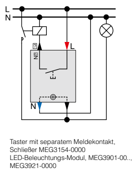
Taster 1-polig mit separatem Meldekontakt für Kontrolllicht
