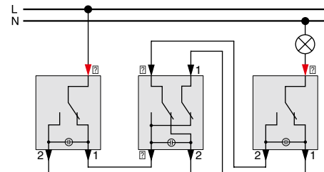
Aus/Wechselschalter mit Orientierungslicht MEG3136-0000
