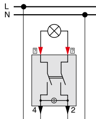
Aus-Kontrollschalter, 2-polig MEG3102-0000
