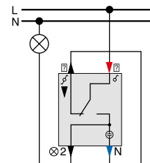
Aus/Wechsel-Kontrollschalter MEG3106-0000
