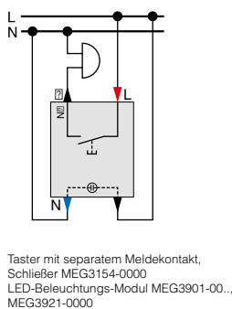
Taster 1-polig mit separatem Meldekontakt für Orientierungslicht
