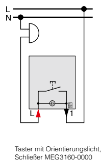
Taster mit Orientierungslicht
