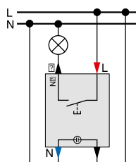
Taster für Card-Schalter mit separatem Meldekontakt und Orientierungslicht, Schließer MEG3754-0000
