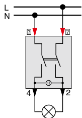
Aus-Kontrollschalter, 2-polig MEG3102-0000
