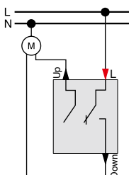
Rolladenschalter MEG3715-0000
